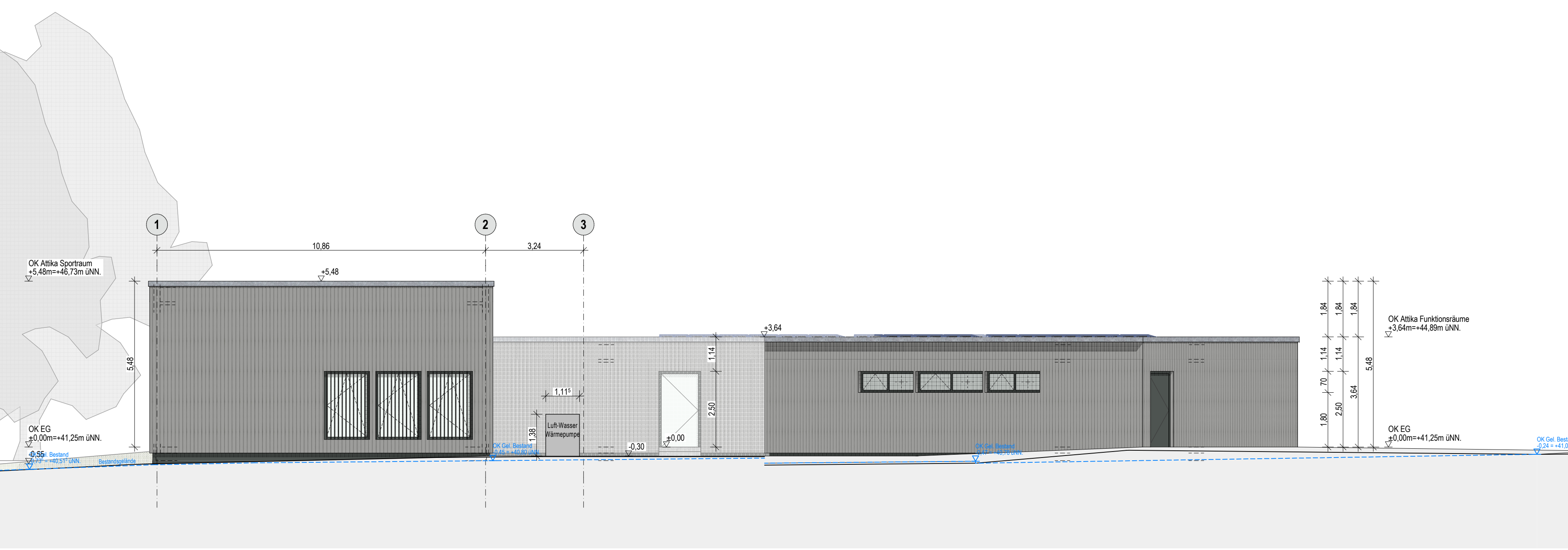
Ansicht Süd-West M 1 | 100
